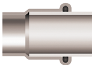
Przekrój połączenia przed zaprasowaniem
