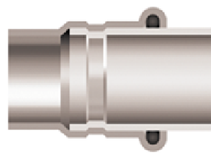
Przekrój połączenia po zaprasowaniu
